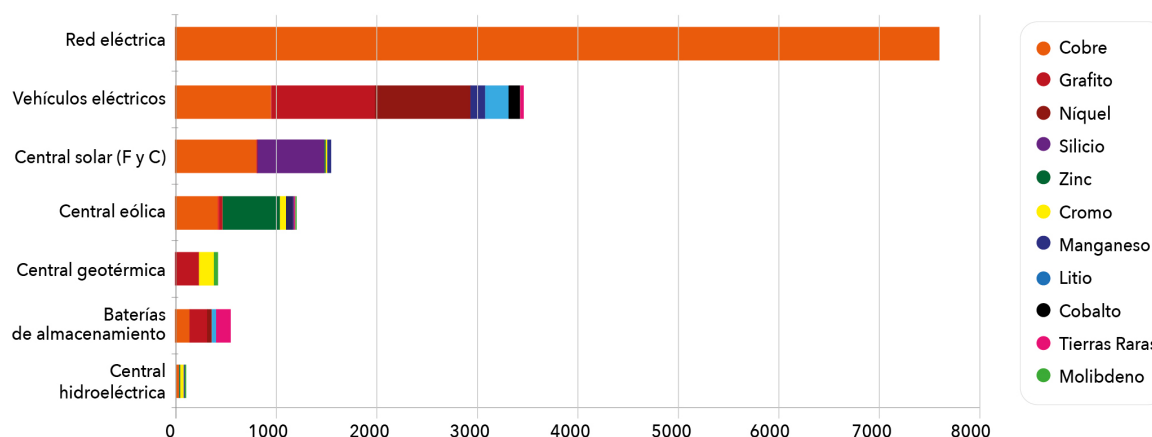
Gráfica 1. ESTIMACIÓN DE LA CANTIDAD DE METALES Y MINERALES NECESARIOS EN LOS DISTINTOS SECTORES DE LA TRANSICIÓN ENERGÉTICA PARA EL AÑO 2040 (SEGÚN EL ESCENARIO DE POLÍTICAS DECLARADAS), EN MILES DE TONELADAS.
